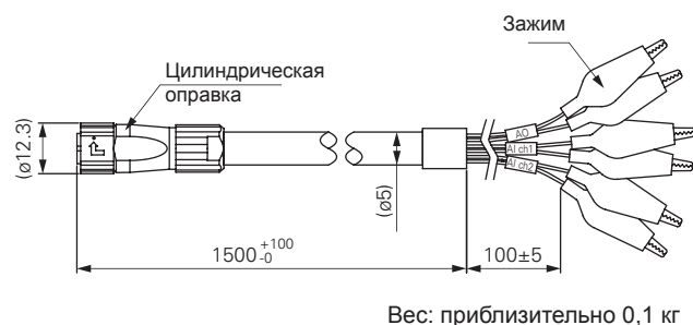
Датчик FLD51 (Большой тип)
