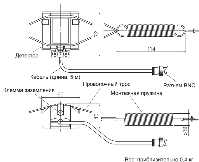
Детектор FLD41 (средний тип)
